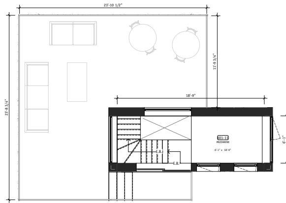
1 PLAN 601 - 6 E ÉTAGE A178 1/8" = 1'-0"
